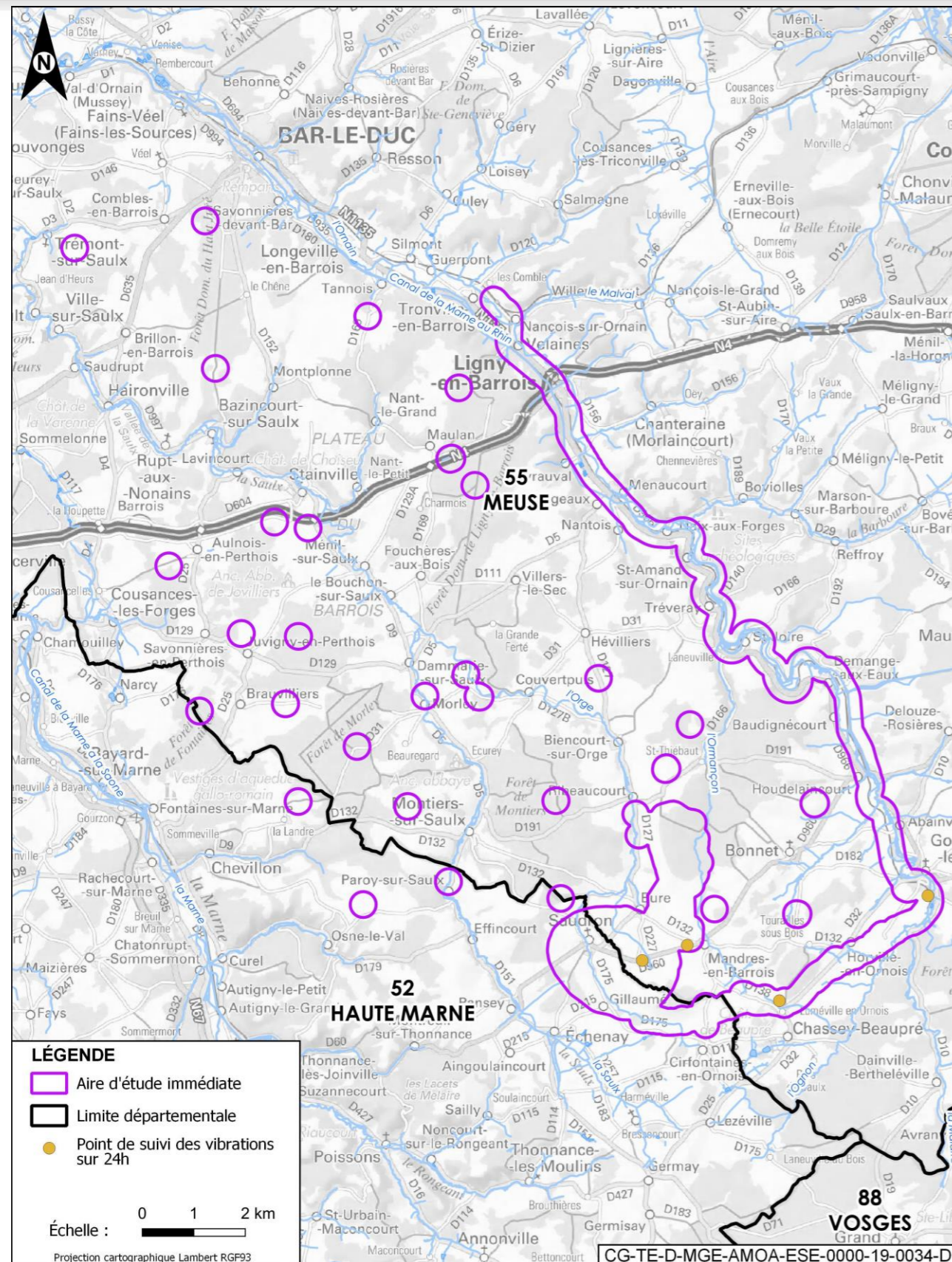
Figure 13-7 Localisation des points de mesures de vibration
