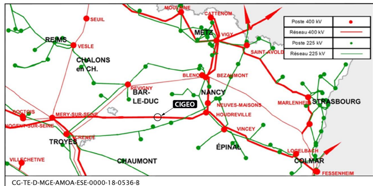
Figure 9-2 Localisation du raccordement électrique du centre de stockage Cigéo sur le réseau 400 kV
