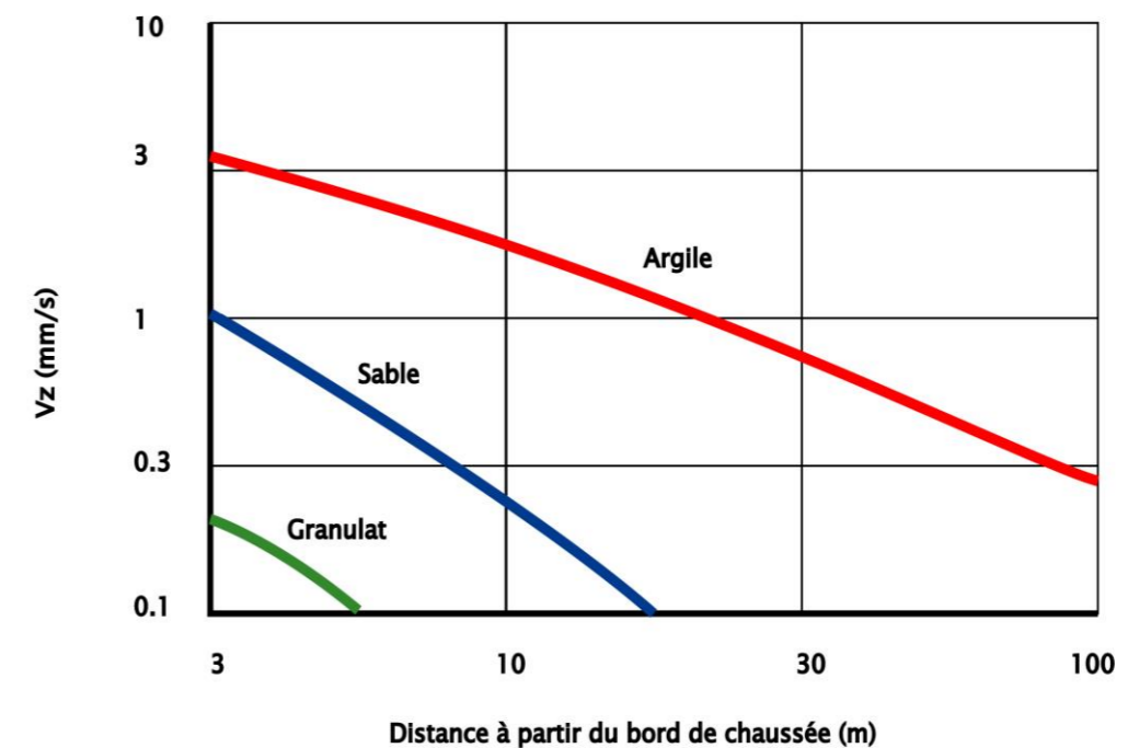
Figure 13-6 Effet de la distance et du type de sol sur la propagation des vibrations
