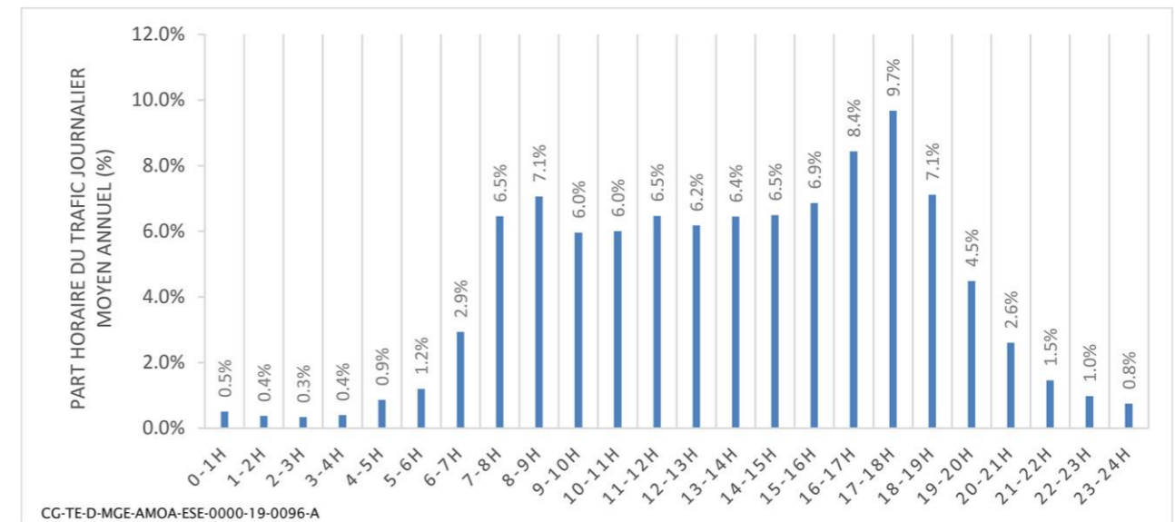
Figure 12-5 Profil horaire moyen « tous véhicules » sur le réseau départemental à proximité du projet global Cigéo
