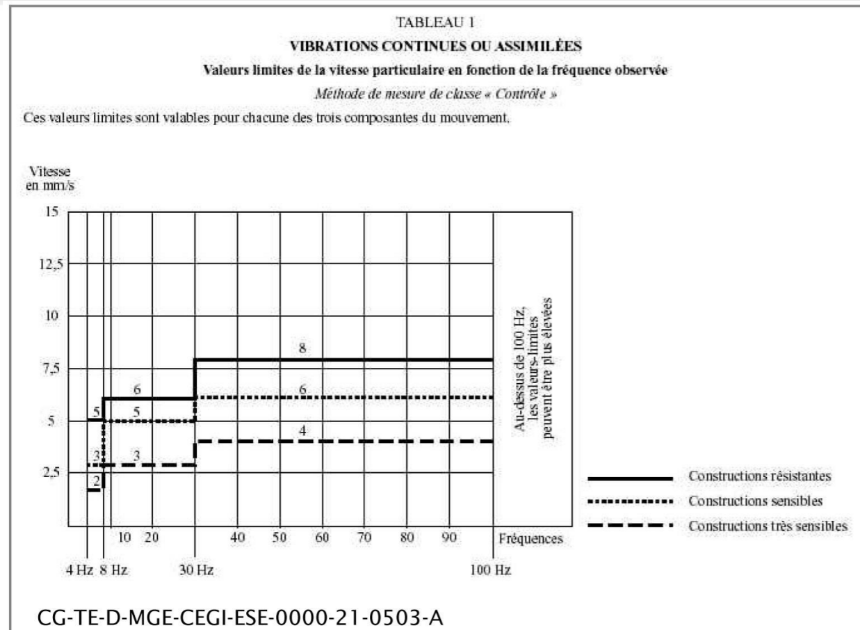
Figure 13-8 Valeurs limites de la vitesse particulière en fonction de la fréquence observée (source : circulaire du 23 juillet 1986 (128))
